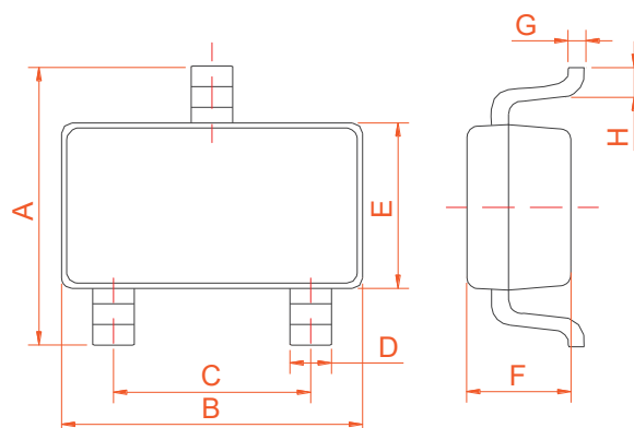
SOT-23-3L
