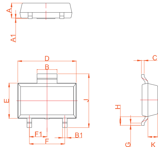
SOT-89-2L
