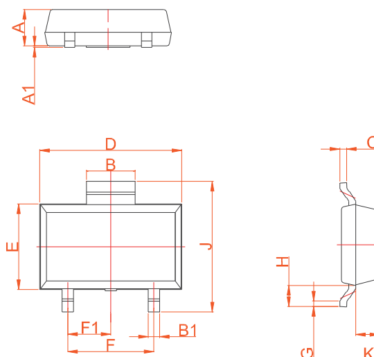
SOT-89-2L
